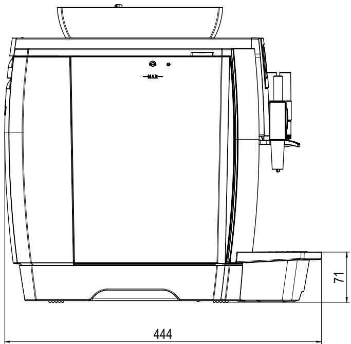
Seitenriss
